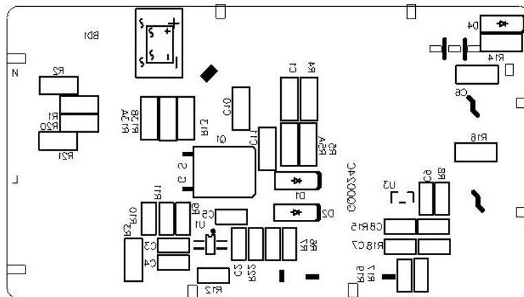
BOTTOM LAYER
